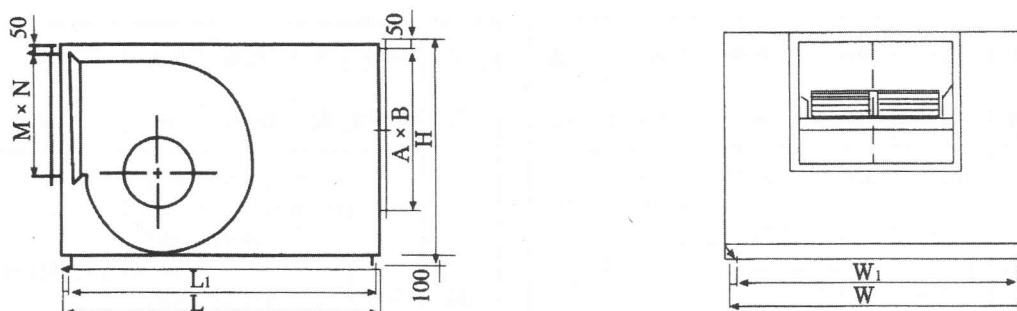
5). DBF-S 型双速低噪声风机箱外形图
